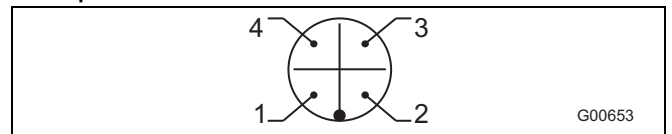
Рис. 44: назначение выводов при подключении через опциональный штекер M12 (вид спереди на контакты)
