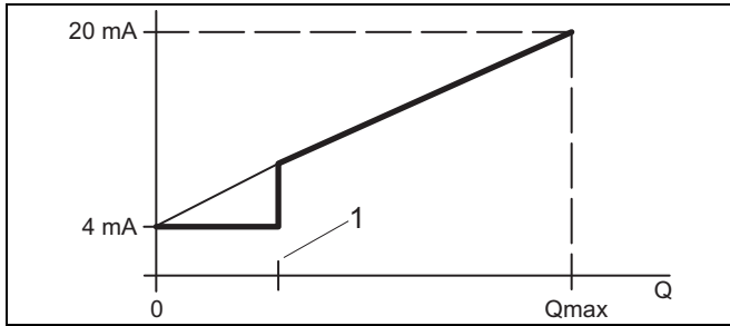
Рис. 28: Токовый выход 1 мин. порог расхода
