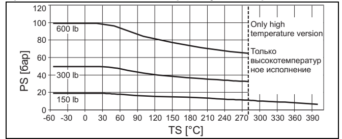
Рис. 16: только высокотемпературное исполнение PS давление (бар) TS температура (°C)
