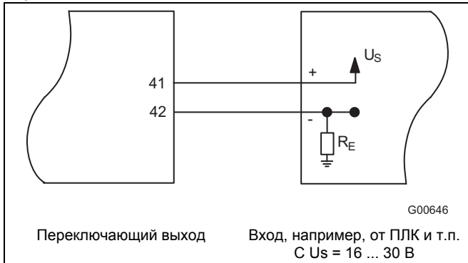
Рис. 27: Электрическое подключение
