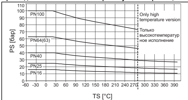
Рис. 15: только высокотемпературное исполнение PS давление (бар) TS температура (°C)
