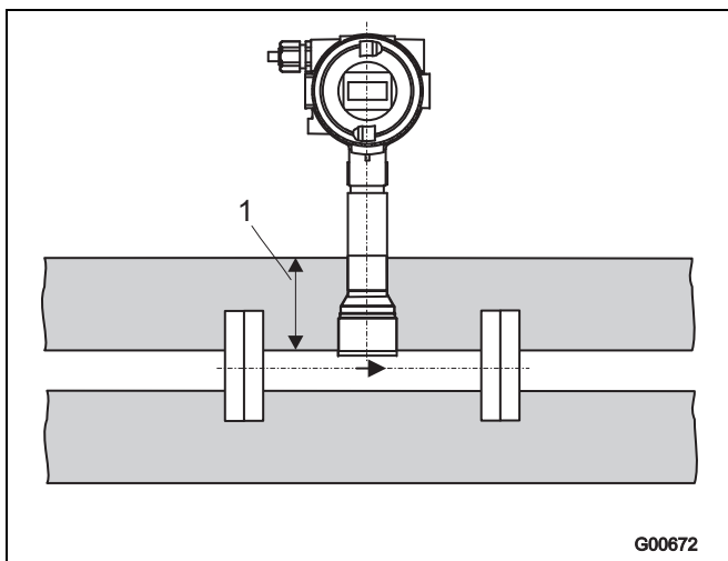
Рис. 6: изоляция расходомера
