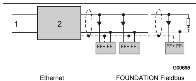
Рис. 35: пример подключения по интерфейсу FOUNDATION Fieldbus
