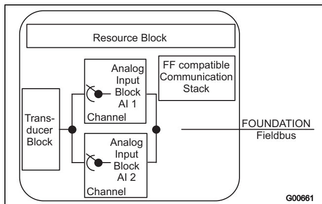
Рис. 34: структура блоков в FOUNDATION Fieldbus
