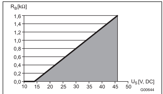
Рис. 25: диаграмма нагрузки токового выхода; нагрузка по питанию
